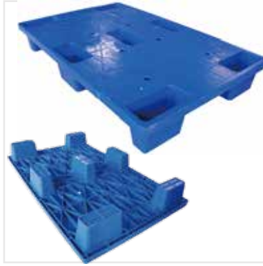
QUA-SFP02 Seven Feet Pallet 1200*800*150mm S.T: 1200kg D.T: 500kg
